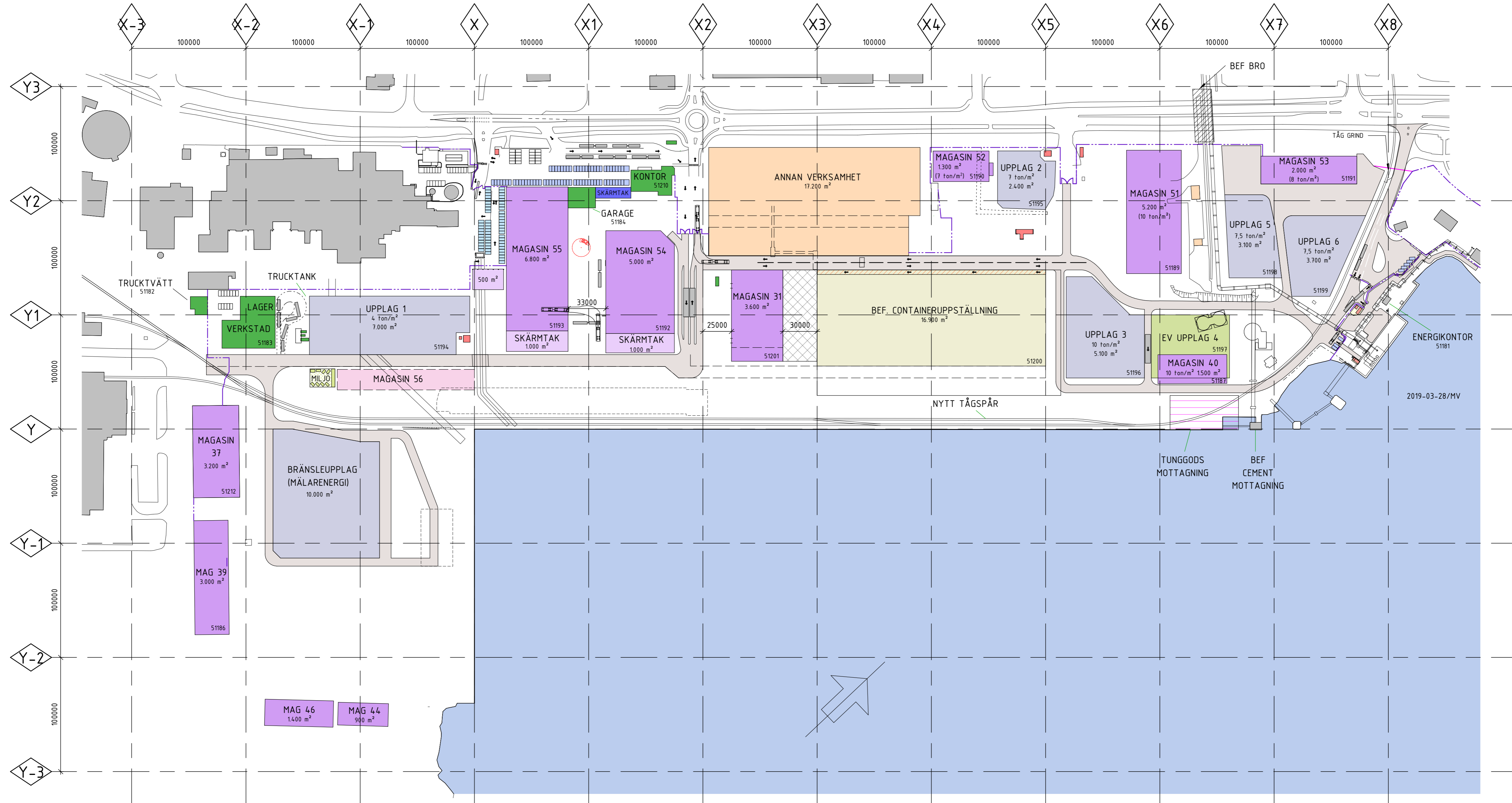
Hamnlayout 2019-09-25 /M. Vestin
